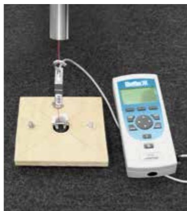
Устройство для «испытания каблуком» Тестирование прочности фиксаторов для ковриков
